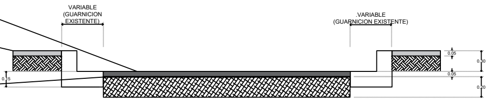
DETALLE CORTE TRANSVERSAL
