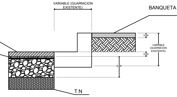
DETALLE DE CORTE
